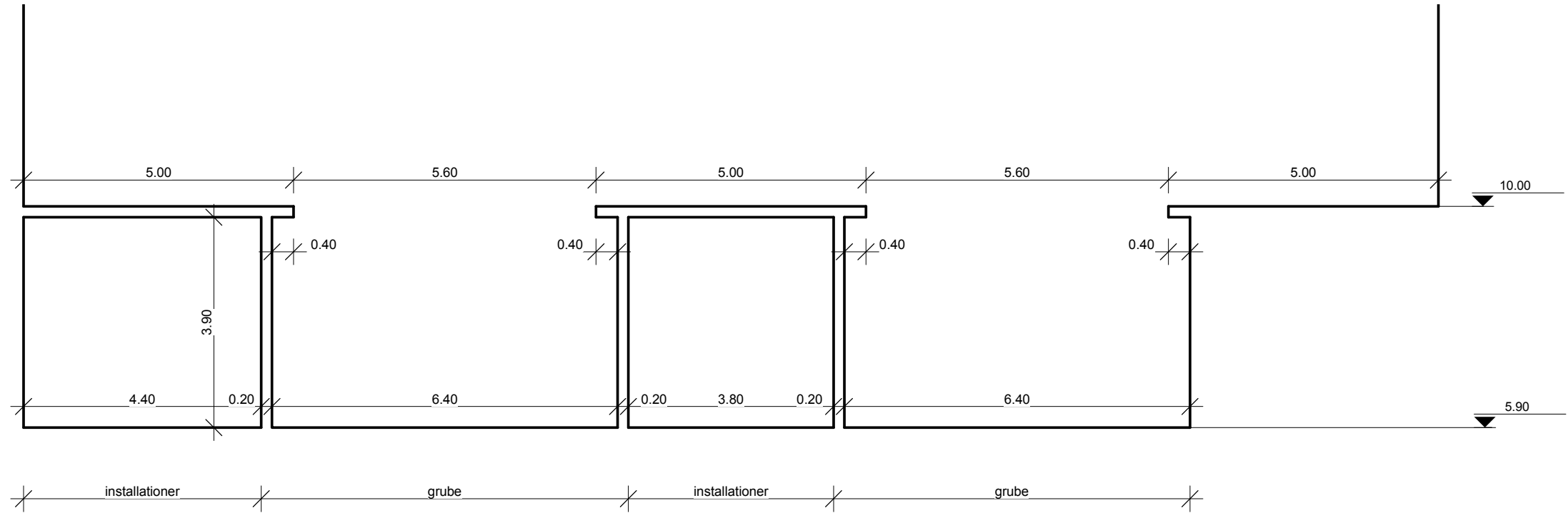
PRINCIPSNIT AA - TVÆRSNIT I MODTAGEHAL 1:100
